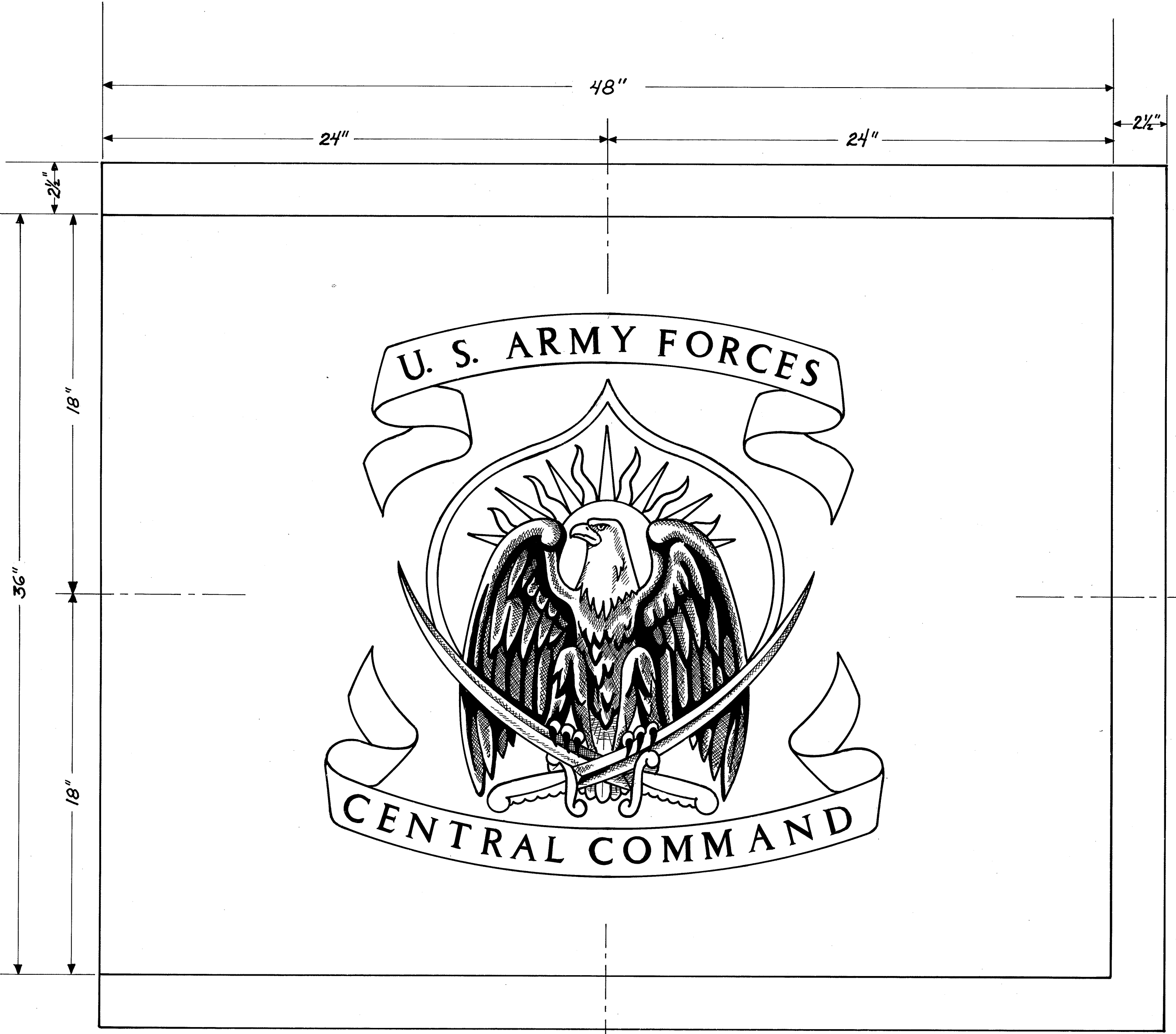
SCALE: 1/4 ACTUAL SIZE OF 3'-0" x 4'-0" FLAG
